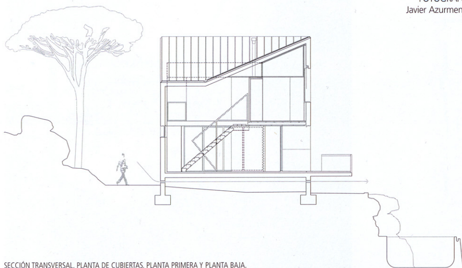
SECCIÓN TRANSVERSAL, PLANTA DE CUBIERTAS, PLANTA PRIMERA Y PLANTA BAJA.
